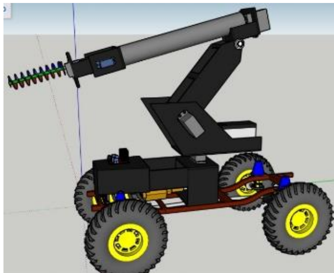
Figura 1. Estructura del robot. Elaboración propia.
