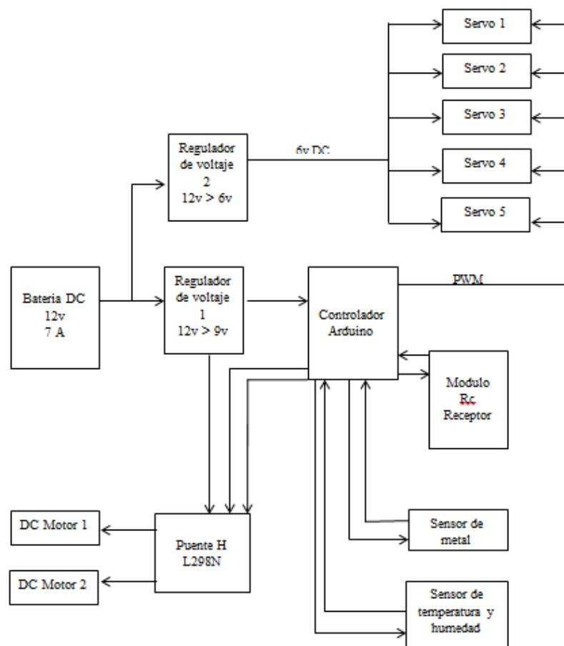
Figura 2. Esquema eléctrico del robot explorador. Elaboración propia.
